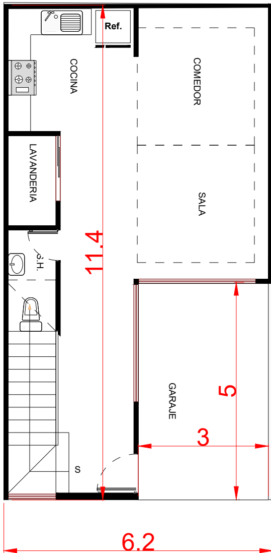
Planta baja
