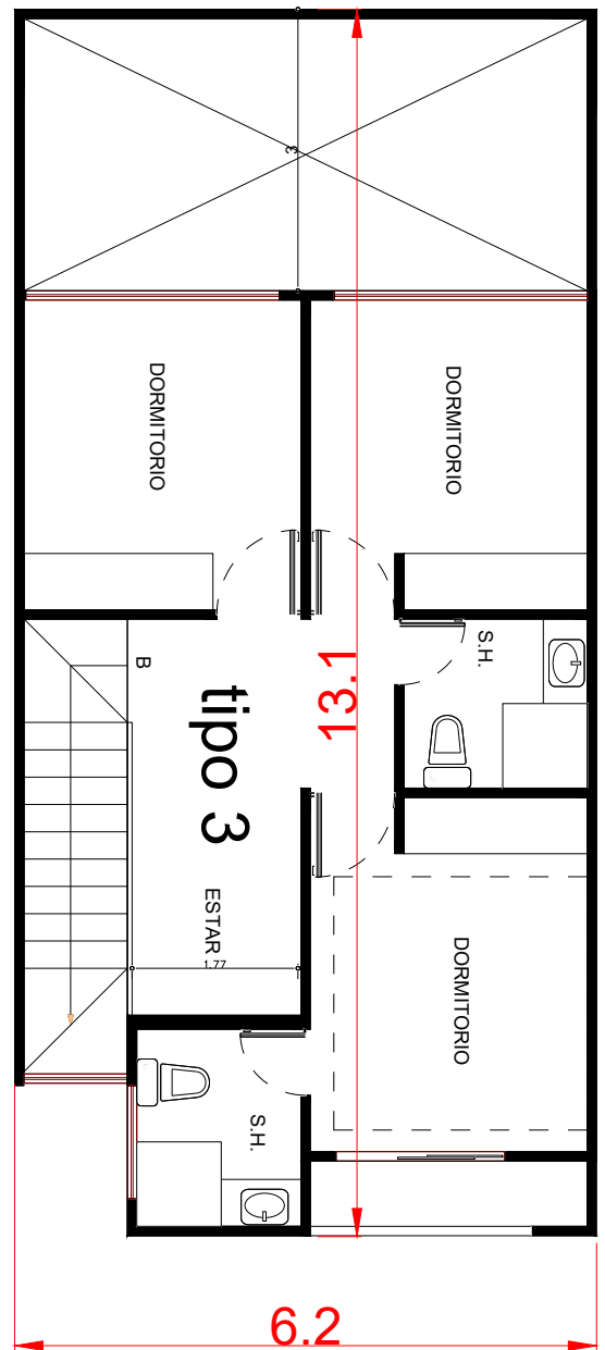
Planta alta
